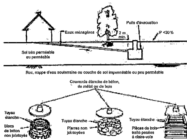
Figure B.17.3 : Le puits d'évacuation
